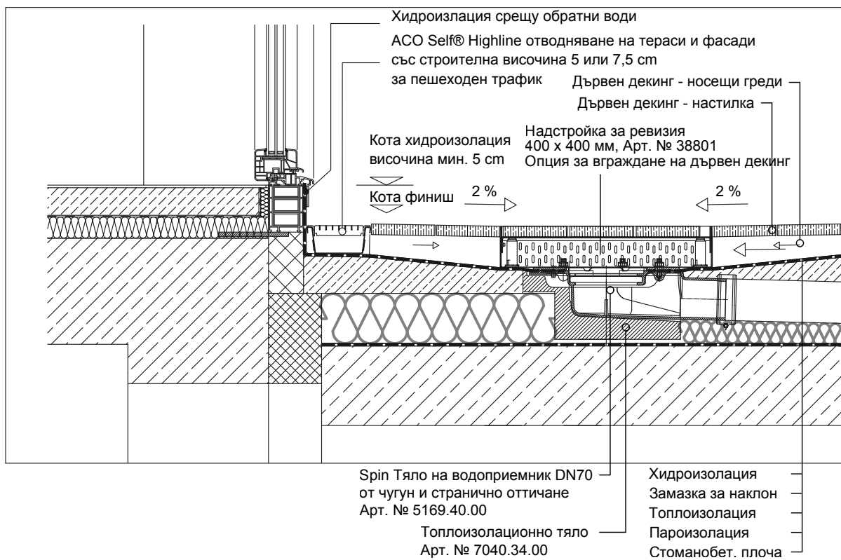
2 ACO Highline в дървен декиннг, водоприемник със странич. заустване и надстройка за ревизия, вариант с топъл покрив 1:10
