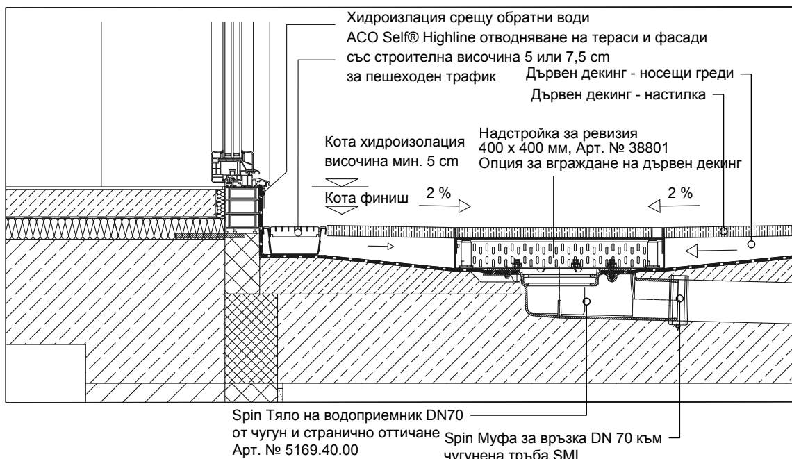
1 ACO Highline в дървен декиннг, водоприемник със странич. заустване и надстройка за ревизия, вариант със студен покрив 1:10
