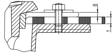
ДЕТАЙЛ С-С 1:2.5
