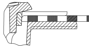
ДЕТАЙЛ С-С 1:2.5
