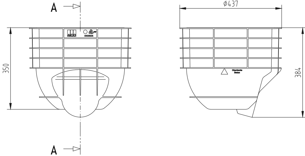
Разрез A-A
