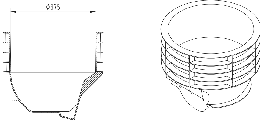
Разрез A-A
