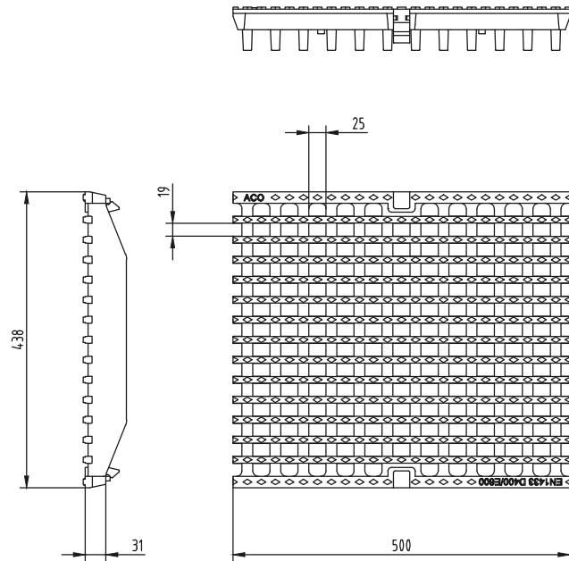
Решетка с надлъжни отвори чугун, клас D400-E600
