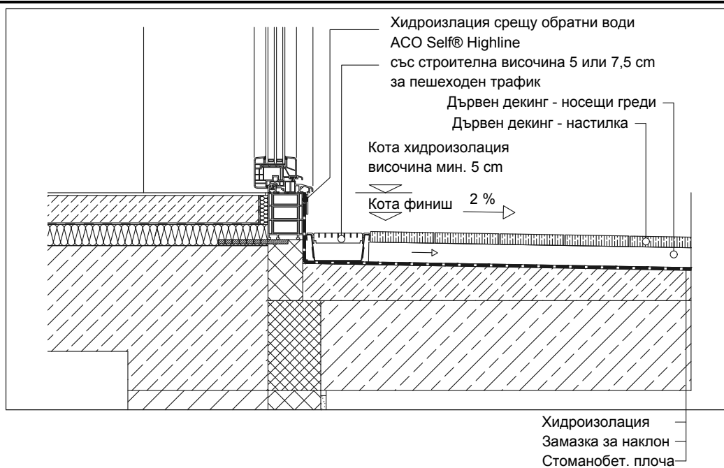
1 Детайл за монтаж на ACO Highline в дървен декинг и странично заустване
