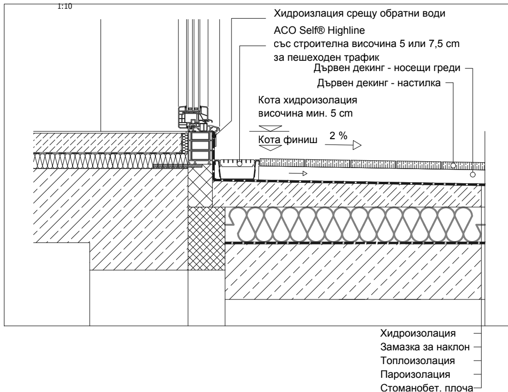
2 Детайл за монтаж на ACO Highline в дървен декинг, стран. заустване и топъл покрив
