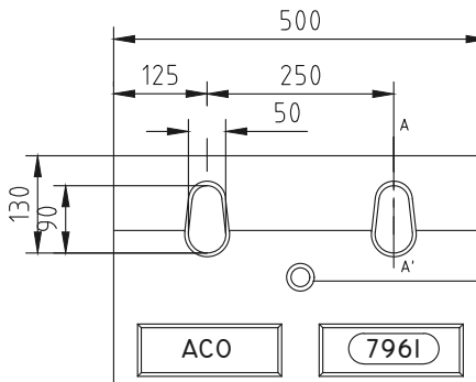
Изглед Отпред
