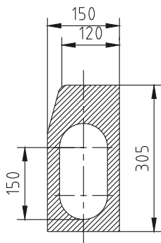
Изглед отстрани
