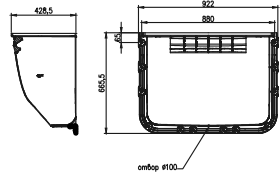
ACO Markant Светлинна шахта 800 x 600 x 400 мм
