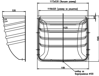
ACO Markant Светлинна шахта 1000 x 1000 x 500 мм
