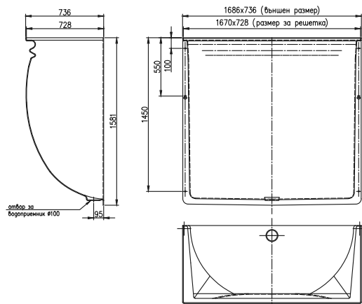
ACO Markant Светлинна шахта със стъклена решетка
