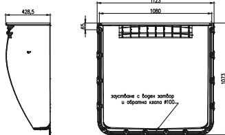
ACO Markant Светлинна шахта 1000 x 1000 x 400 мм
