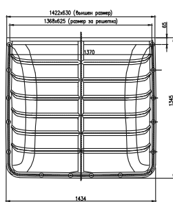
ACO Markant Светлинна шахта 1250 x 1300 x 600 мм
