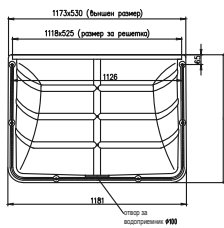
ACO Markant Светлинна шахта 1000 x 800 x 500 мм
