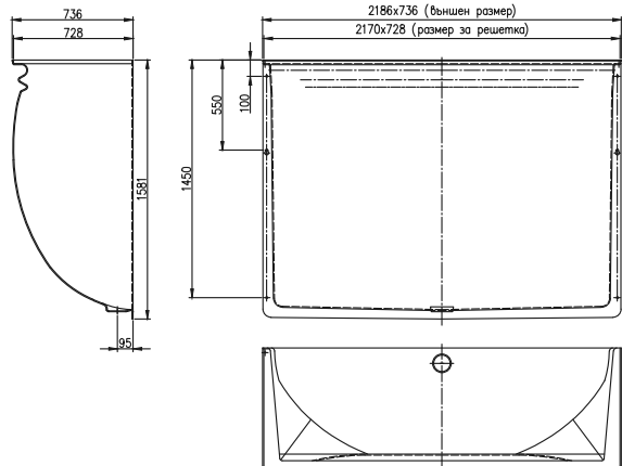
ACO Markant Светлинна шахта 2000 x 1500 x 700 мм
