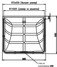
ACO Markant Светлинна шахта 800 x 800 x 500 мм
