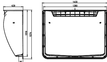
ACO Markant Светлинна шахта 1250 x 1000 x 400 мм
