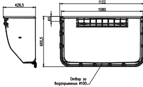
ACO Markant Светлинна шахта 1000 x 600 x 400 мм
