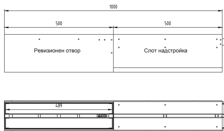
Слот надстройка за ревизия с центричен слот клас D400
