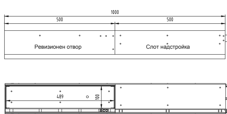
Слот надстройка за ревизия с ексцентричен слот клас C250
