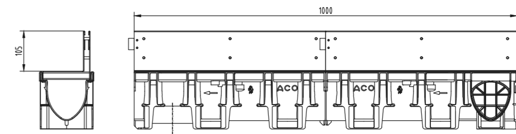
SlotDrain 100 Слот надстройка с ексцентричен слот и улей ExtraDrain 100
