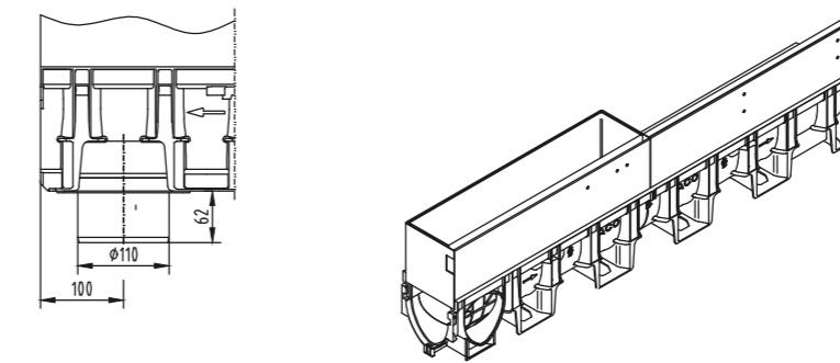
SlotDrain 100 Слот надстройка за ревизия с ексцентричен слот и водосъбирателна шахта ExtraDrain 100
