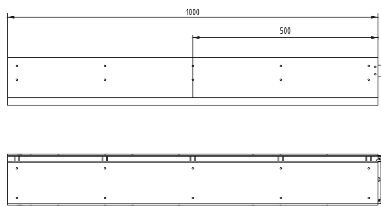
SlotDrain Слот надстройка с ексцентричен слот за улей, клас C250
