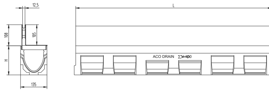
SlotDrain 100 Слот надстройка с ексцентричен слот и улей MultiDrain V 100 тип 0.0 до 20.0
