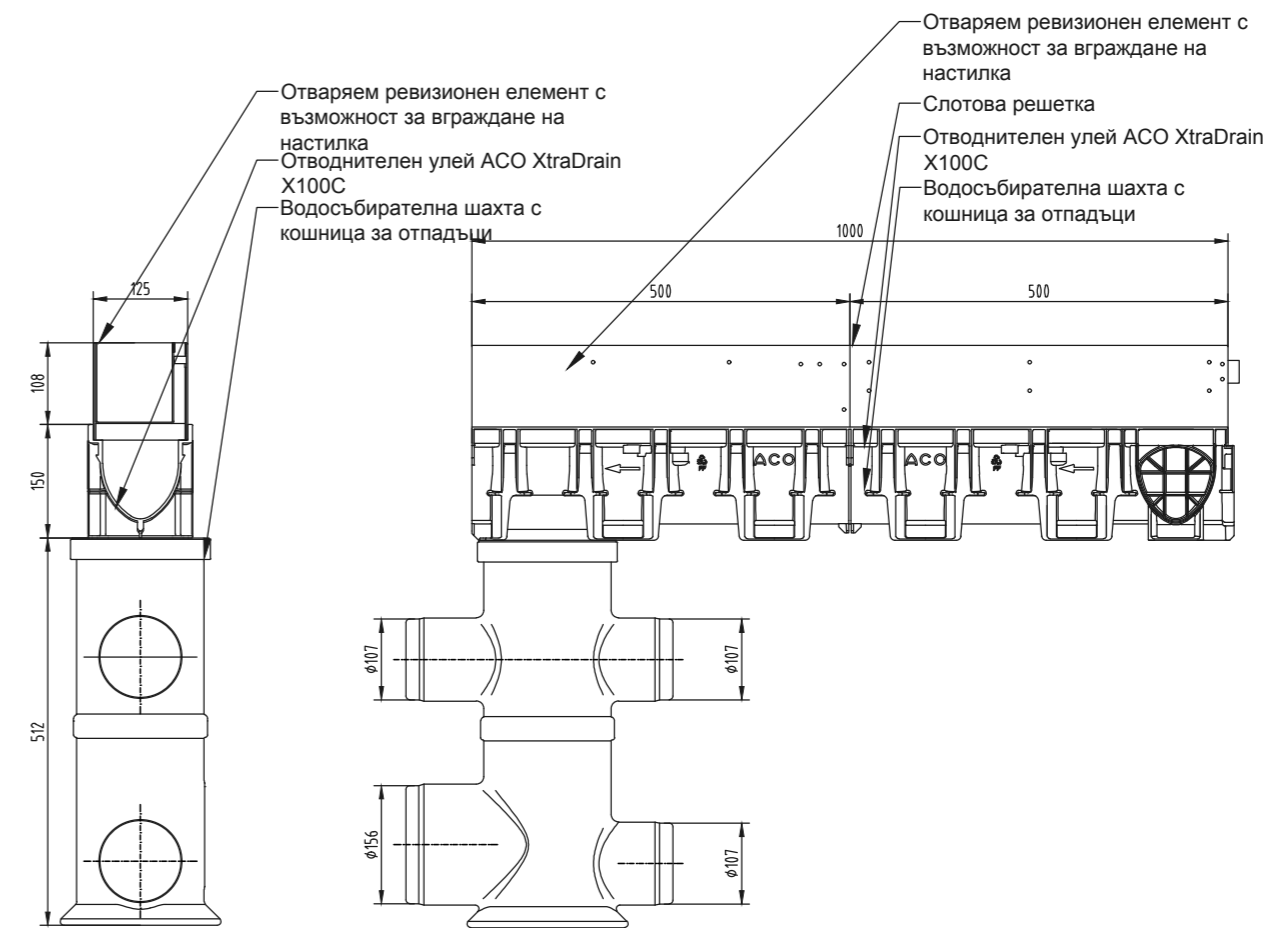
SlotDrain 100 Слот надстройка за ревизия с ексцентричен слот и водосъбирателна шахта ExtraDrain 100
