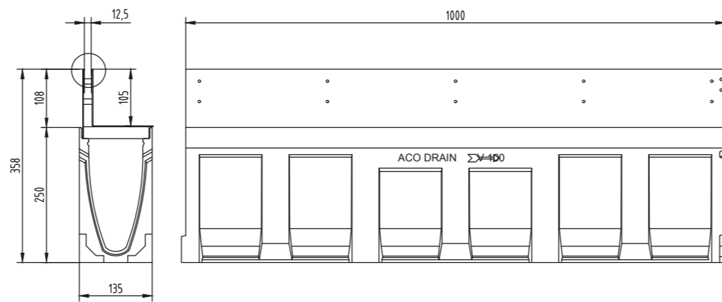
SlotDrain 100 Слот надстройка с ексцентричен слот и улей MultiDrain V 100 тип 0.0 до 20.0
