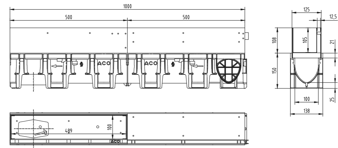
SlotDrain 100 Слот надстройка за ревизия с ексцентричен слот и улей ExtraDrain 100
