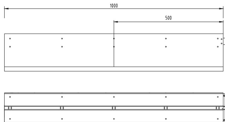
Слот надстройка с центричен слот за улей, клас D400
