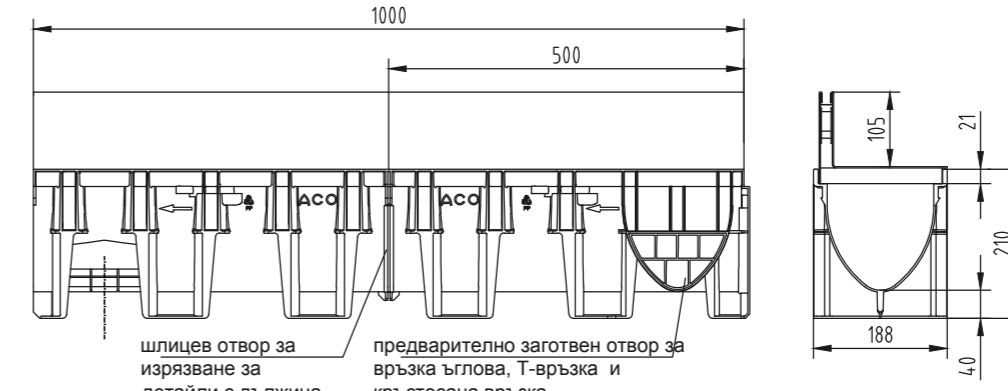
SlotDrain 100 Слот надстройка с ексцентричен слот и улей ExtraDrain 100
