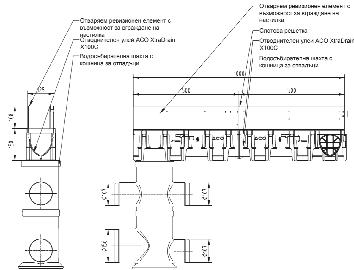
SlotDrain 100 Слот надстройка за ревизия с ексцентричен слот и водосъбирателна шахта ExtraDrain 100
