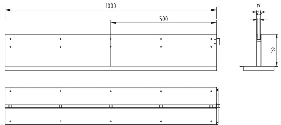
Слот надстройка за ревизия с ексцентричен слот клас C250
