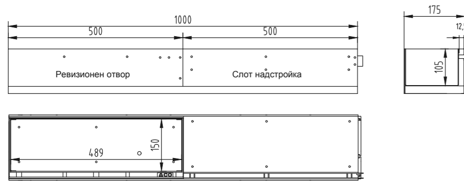
Слот надстройка за ревизия с ексцентричен слот клас C250
