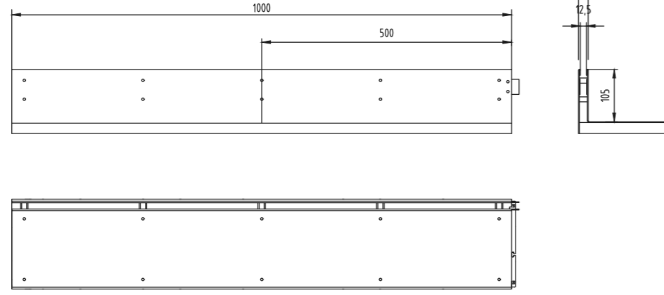
SlotDrain Слот надстройка с ексцентричен слот за улей, клас C250
