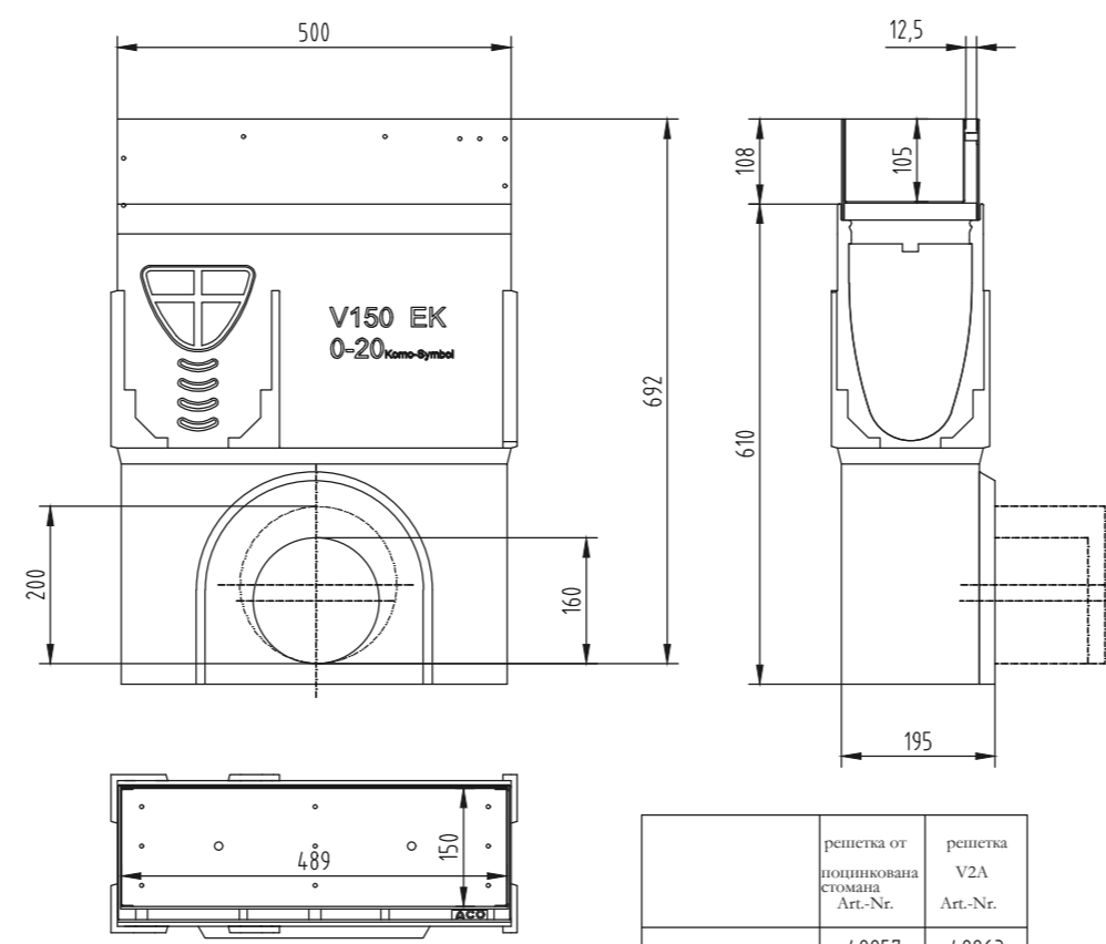
SlotDrain Слот надстройка за ревизия с ексцентричен слот и водосъбирателна шахта MultiDrain V 150
