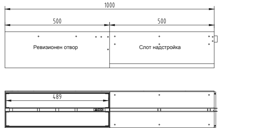
Слот надстройка за ревизия с центричен слот клас D400
