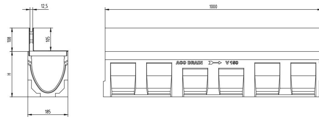
SlotDrain 100 Слот надстройка с ексцентричен слот и улей MultiDrain V 150 тип 0.0 до 20.0
