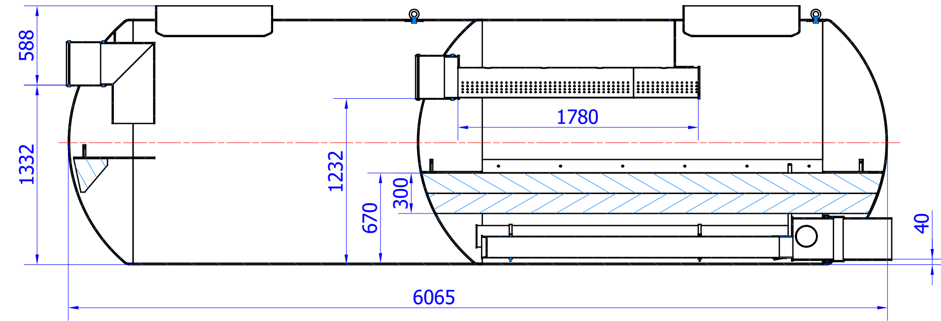
A-A ( 1 : 30 )
