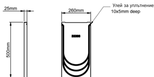
TramDrain 200 челна плоча
