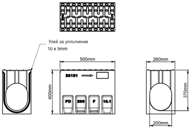
TramDrain 200 отводнителен улей 500mm LG
