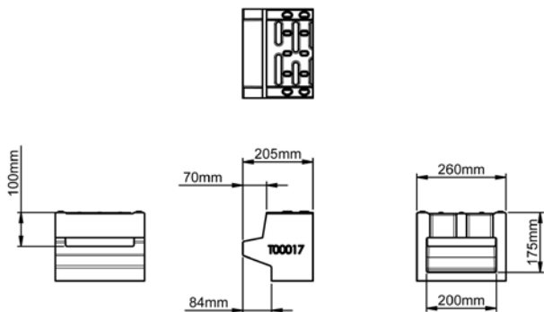
TramDrain 200 релсова връзка
