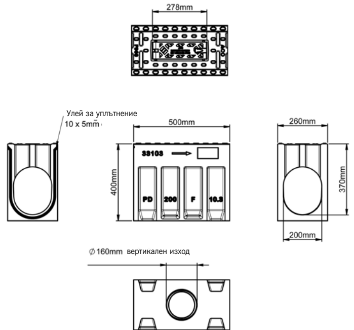
TramDrain 200 ревизионен елемент 500mm LG
